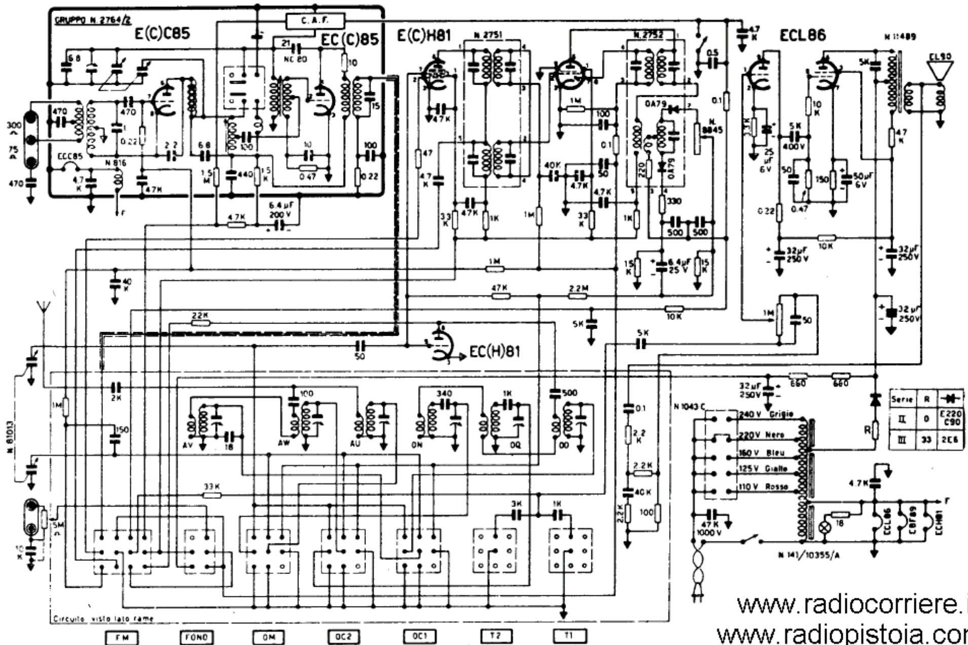
GELOSO - MODD. G.3401/2 - G.3451/2
