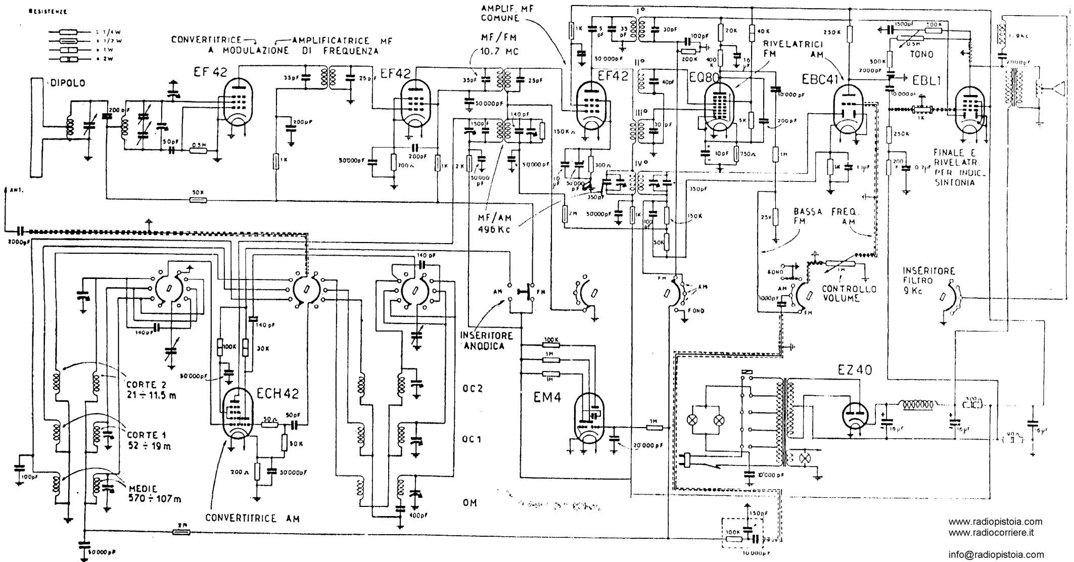
SIEMENS RADIO - Ricevitore AM/FM mod. 841 - A modulazione d'ampiezza: medie e due corte, a modulazione di frequenza: gamma da 88 a 108 megacicli. Media frequenza FM a 10,7 megacicli, media frequenza AM a 469 kc. ECH42 solo per AM.
