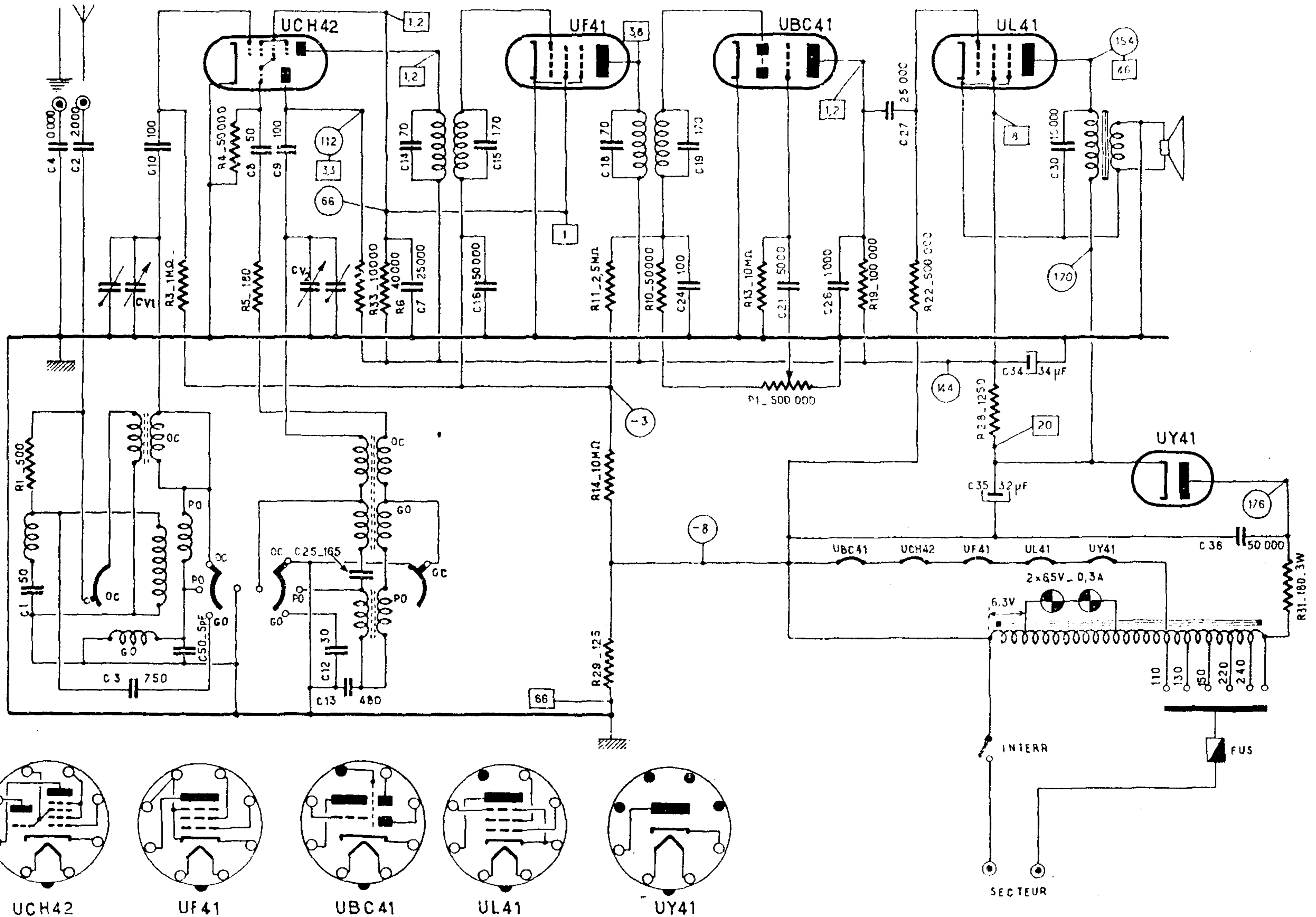
Schéma général du récepteur D925.
